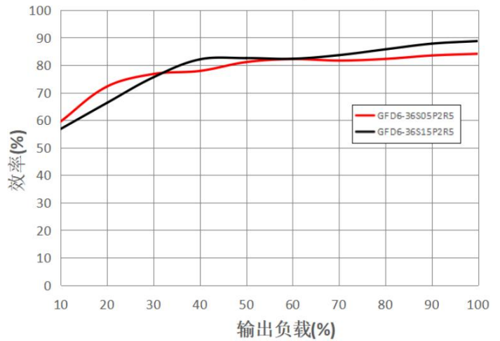
效率VS输出负载 (Vin=48V)
